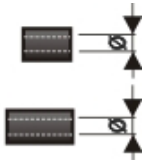
Distanzhülse für Gewindestangen Spacer for threaded rods
